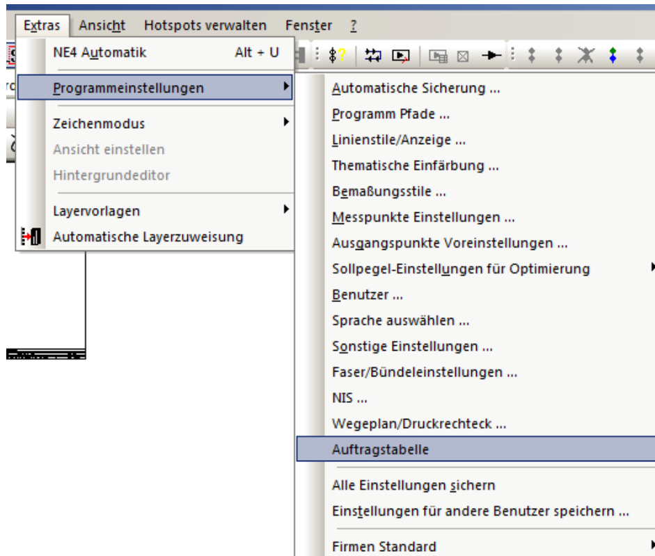
Bild 3: Menüstruktur
